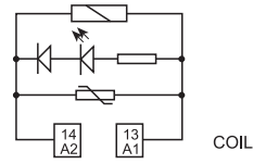
Beispiel: AC
