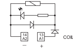
Beispiel: DC
