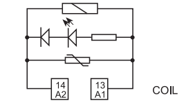
Beispiel: AC
